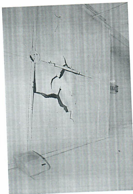
Фото 8. Помещение первого этажа.
