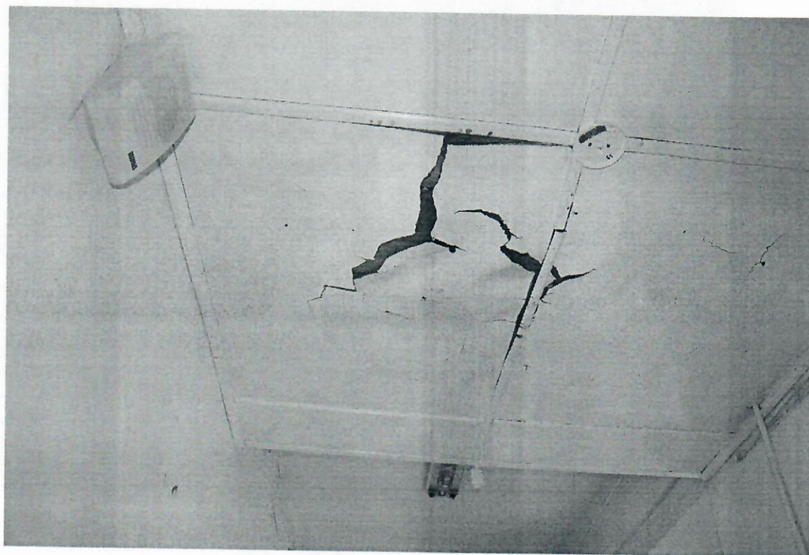
Фото 25. Трещины на потолке.
