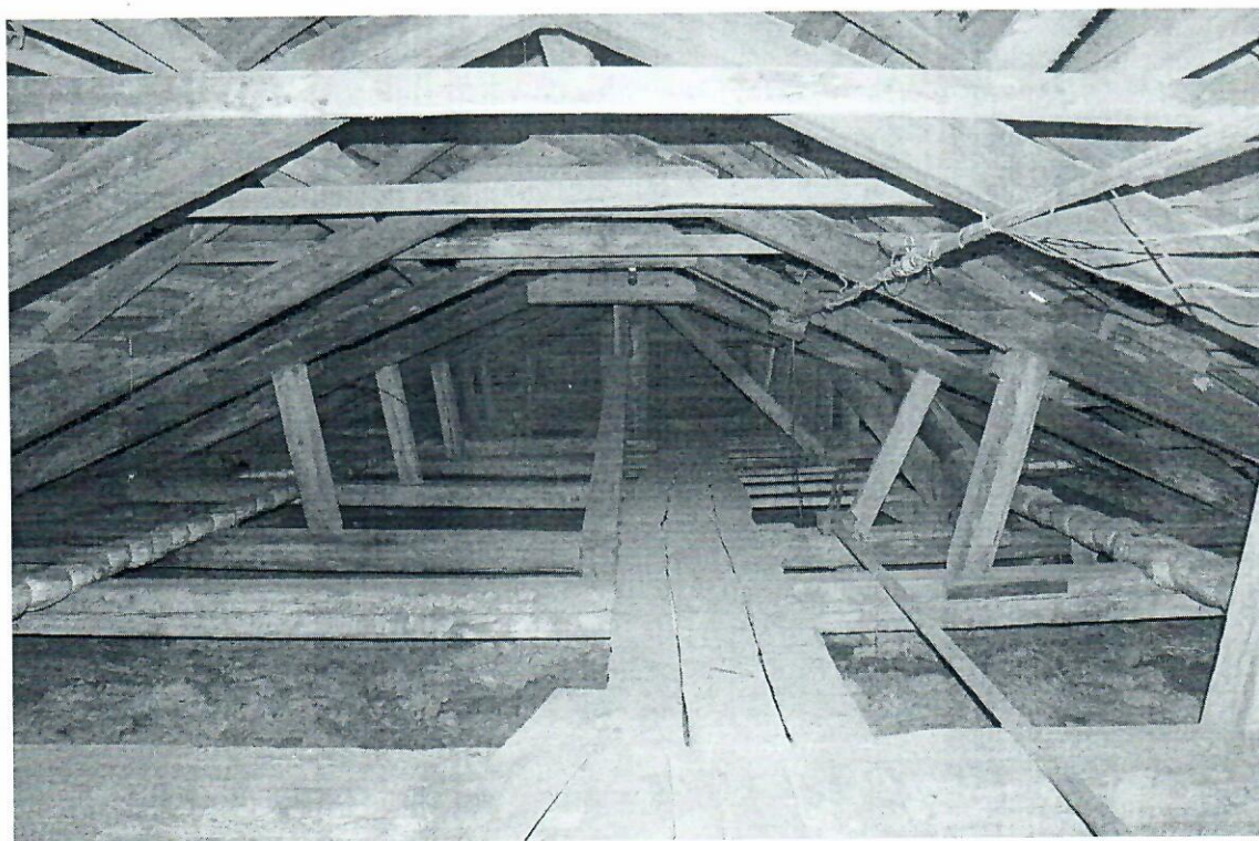
Фото 35. Состояние стропильных конструкций.
