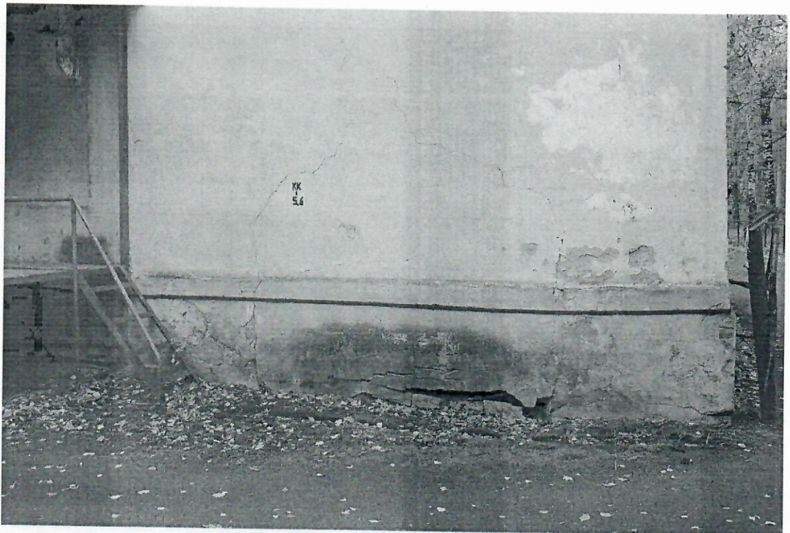
Фото 5. Состояние цокольной части.
