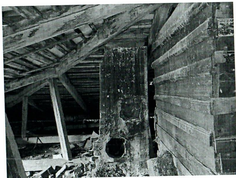
Фото 83. Состояние элементов стропильной системы и печи.
