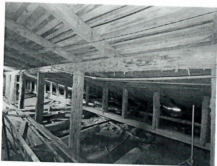
Фото 86. Состояние элементов стропильной системы.
