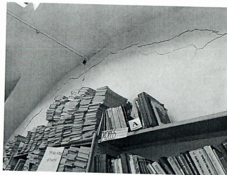
Фото 52. Состояние стен.
