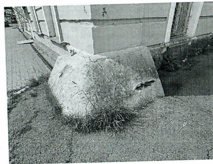
Фото 9. Состояние цокольной части.
