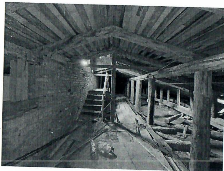
Фото 87. Состояние элементов стропильной системы.
