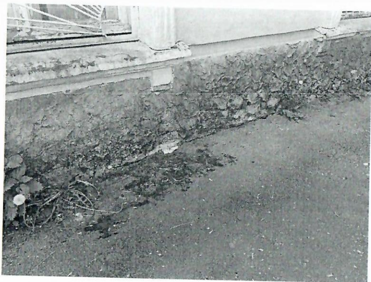
Фото 10. Состояние цокольной части.
