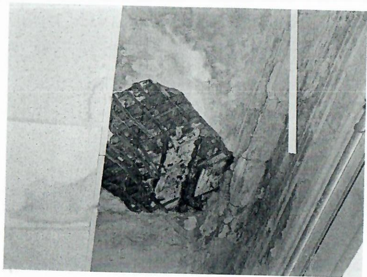
Фото 66. Состояние потолка.
