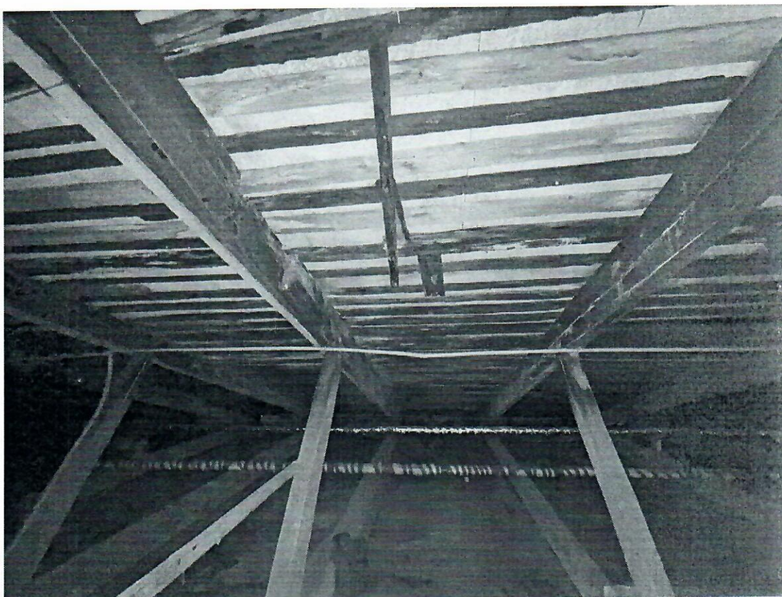
Фото 56. Состояние элементов стропильной системы.
