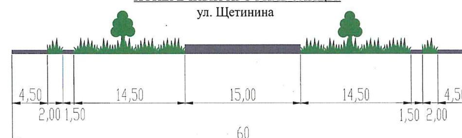
ПОПЕРЕЧНЫЙ ПРОФИЛЬ УЛИЦЫ:
