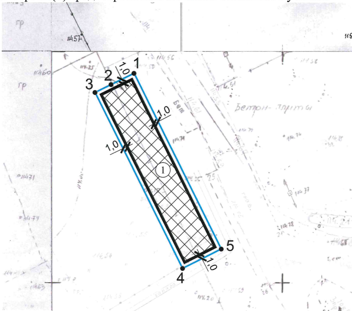
Ситуационный план
